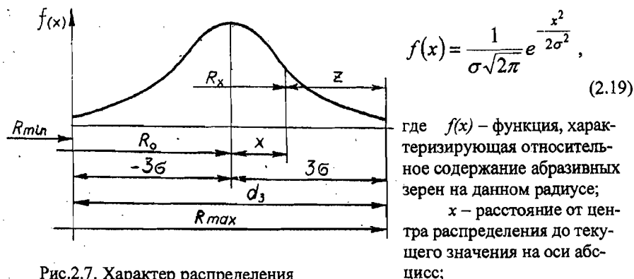
Рис.2.7. Характер распределения абразивных зерен по радиусу камня
