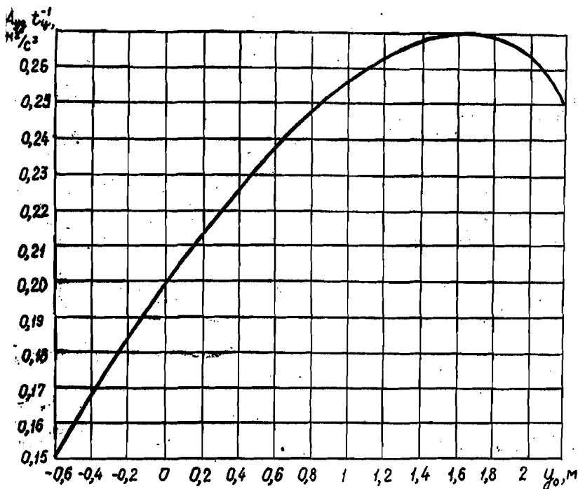
Рис. 1.19. Зависимость A_{y_0} t_u^{-1} = f(y_0) для барабана диаметром 5 м при \omega = 0,28 \omega_{кр}
