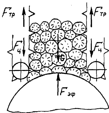
Рис.2.10. Схема усилий в шахте цепного дефибрера
