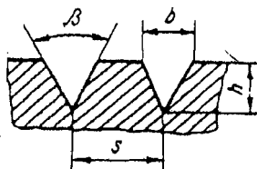
Рис.2.5. Конфигурация поверхности дефибрерного камня после насечки
