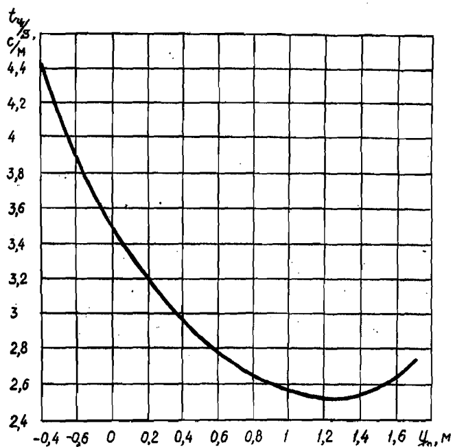
Рис. 1.8. Зависимость t_y S^{-1} = f(y_o) для барабана диаметром 3,85 м при \omega = 0,28 \omega_{кр}
