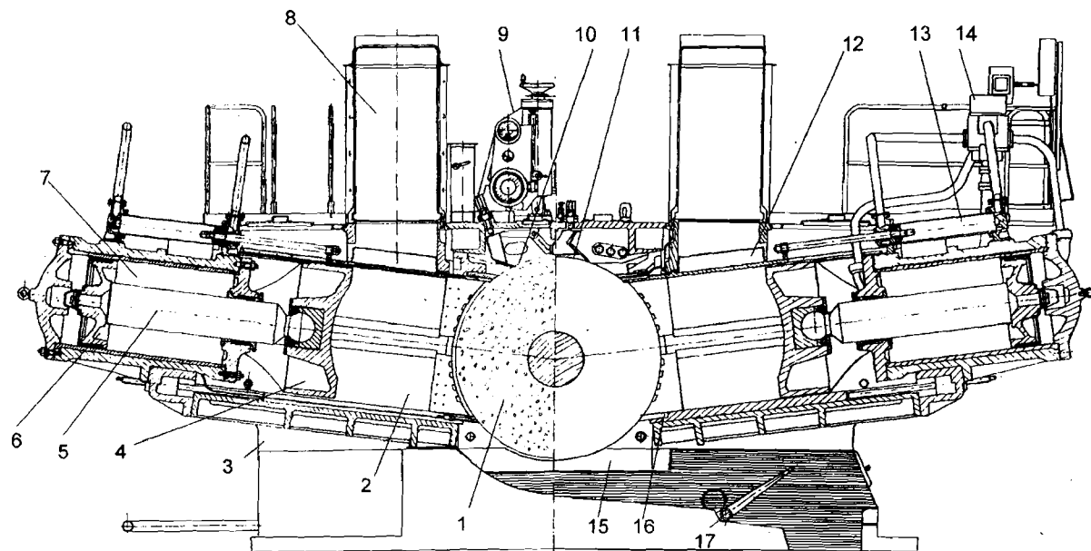
Рис.2.15. Двухпрессовый гидравлический дефибрер: 1-дефибрерный камень; 2- загрузочная камера; 3-корпус с фундаментальными плитами; 4-башмак; 5-шток; 6-поршень; 7-гидроцилиндр; 8-загрузочная шахта; 9-ковочный аппарат; 10, 11-шаберы; 12-шибер; 13-гидроцилиндр шибера; 14-гидравлическая система; 15-ванна; 16-гребенка; 17-переливная перегородка
