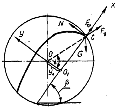
Рис. 1.3. Схема к определению допустимой скорости вращения барабана
