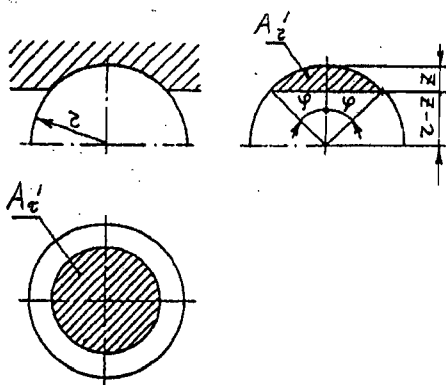
Рис.2.8. Проекция поверхности контакта абразивного зерна с древесиной
