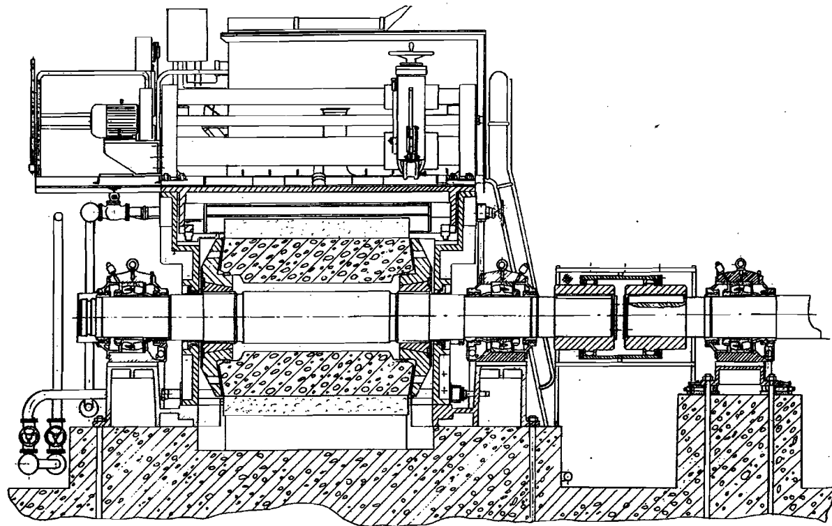
Рис.2.16. Двухпрессовый гидравлический дефибрер (разрез вдоль оси камня)
