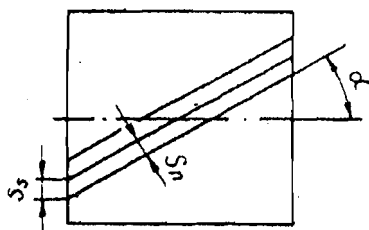
Рис.2.4. Расположение зубьев на поверхности шарошки
