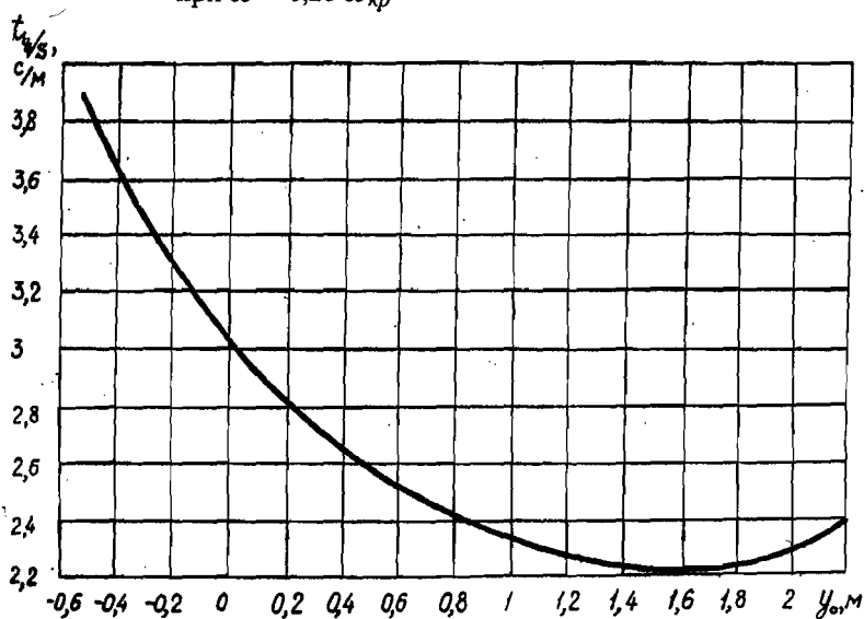
Рис. 1.9. Зависимость t_y S^{-1} = f(y_o) для барабана диаметром 5 м при \omega = 0,28 \omega_{кр}
