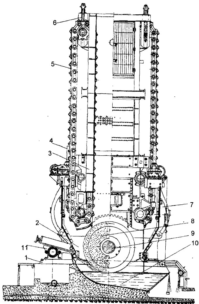
Рис.2.14. Цепной дефибрер: 1-фундаментная плита; 2-неподвижная станина; 3-подвижная шахта; 4-механизм подъема шахты; 5-рабочая цепь; 6-механизм подъема шахты; 6-механизм натяжения рабочей цепи; 7-механизм привода рабочих цепей; 8-дефибрерный камень; 9-вал; 10-ванна; 11-ковочный аппарат
