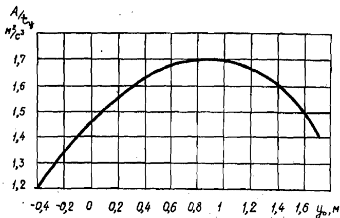
Рис. 1.10. Зависимость At_y^{-1} = f(y_0) для барабана диаметром 3,85 м при \omega = 0,28 \omega_{кр}
