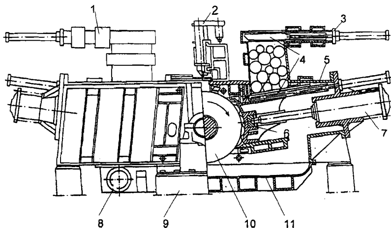
Рис.2.17. Двухпрессовый дефибрер фирмы «Valmet», работающий под давлением: 1-загрузочная камера; 2-аппарат для насечки камня; 3-крышка загрузочной камеры; 4-загрузочный люк; 5-крышка; 6-башмак; 7-прижимной цилиндр; 8-выход массы; 9-фундамент; 10-дефибрерный камень; 11-ванна для массы
