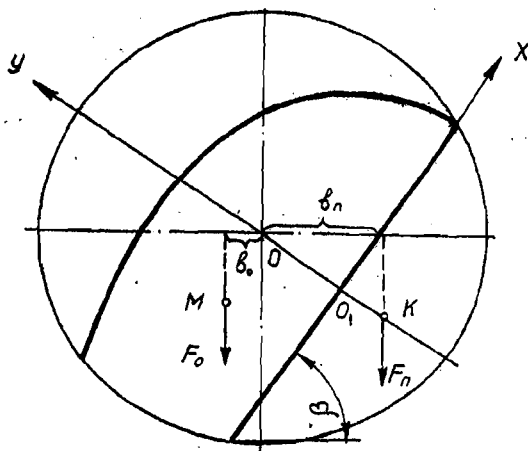
Рис. 1.5. Поперечное сечение участка барабана
