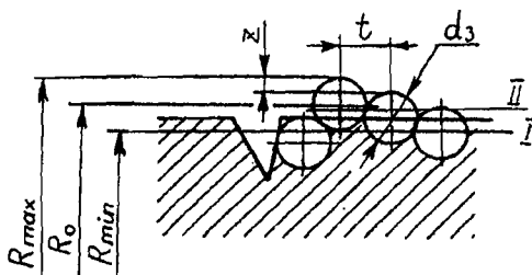
Рис.2.6. Схема распределения абразивных зерен в камне
