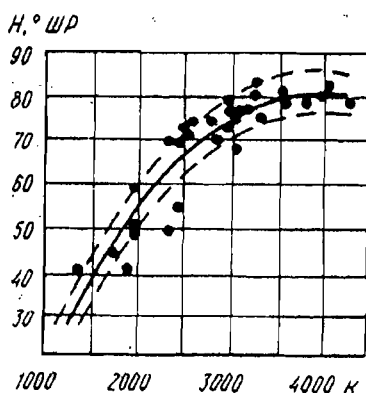
Рис.2.3.Зависимость степени помола древесной массы N (°ШР) от числа циклов нагружений K
