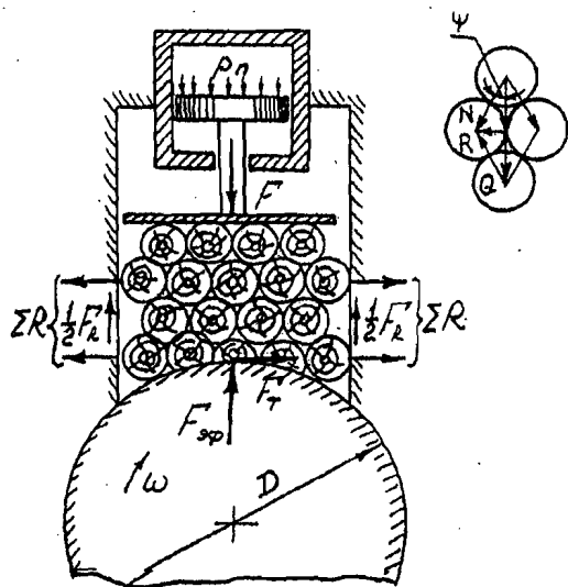
Рис.2.9. Схема усилий в шахте прессового дефибрера
