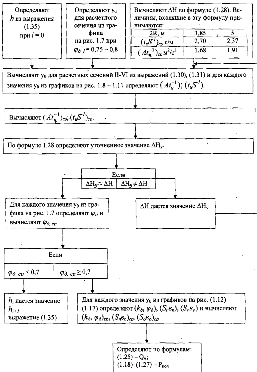
Рис. 1.20. Порядок определения h , Q_m , P_{пол}
