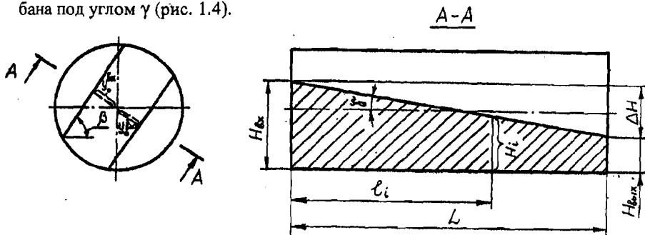
Рис. 1.4. Расположение плоскости обрушения в барабане непрерывного действия
