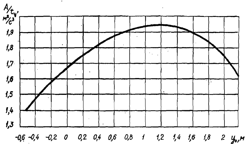
Рис. 1.11. Зависимость At_y^{-1} = f(y_0) для барабана диаметром 5 м при \omega = 0,28 \omega_{кр}
