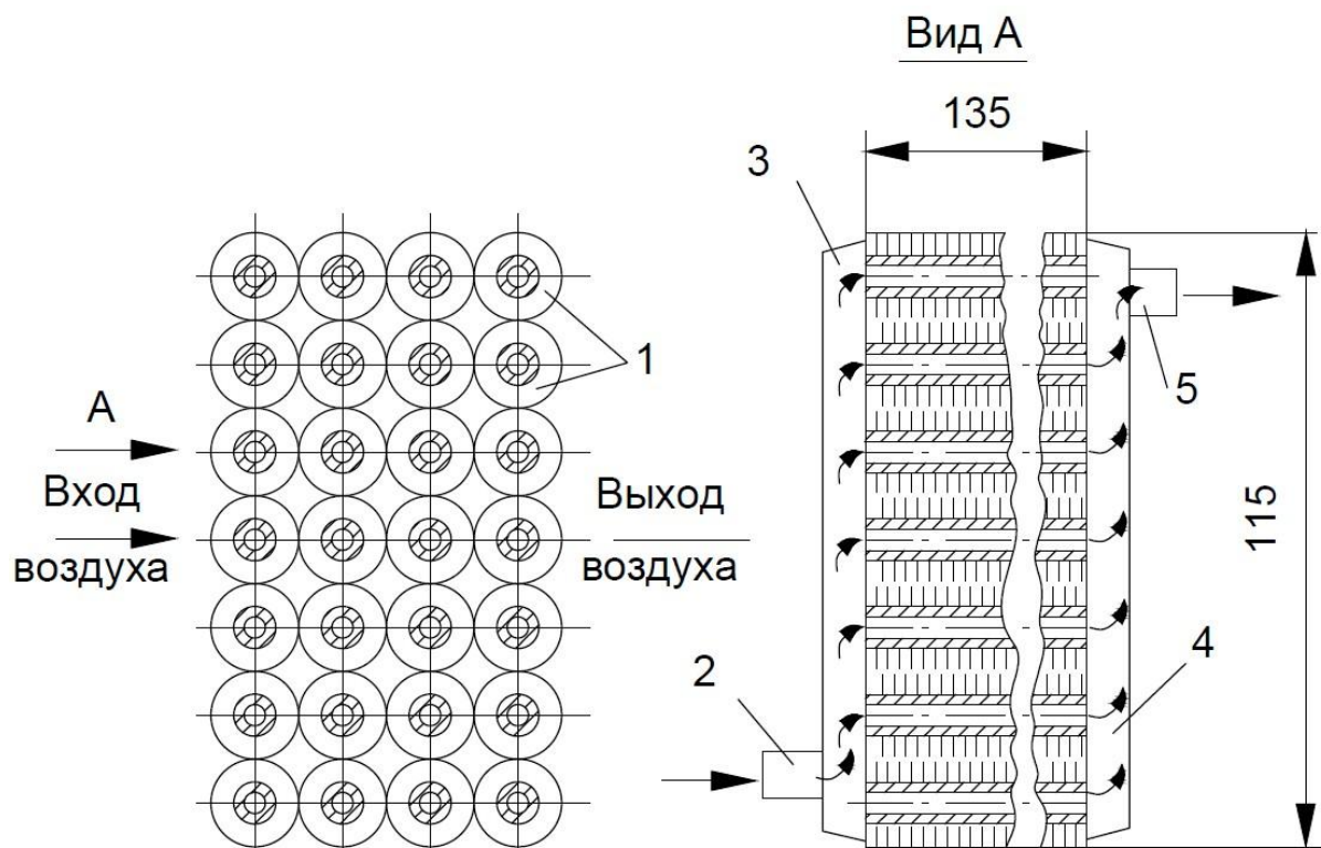
Рис. 2. Схема рабочего участка:
