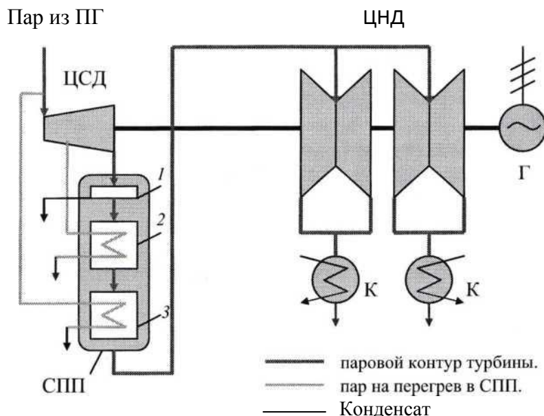
Рис. 3.17. Принципиальная тепловая схема турбины АЭС для работы на влажном паре: 1 - сепаратор влаги; 2, 3 - ступени перегревателя пара
