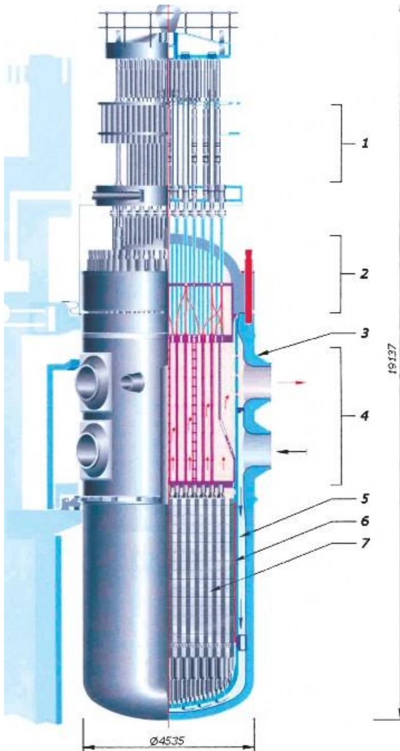
Рис. 3.9. Реактор ВВЭР-1000:
