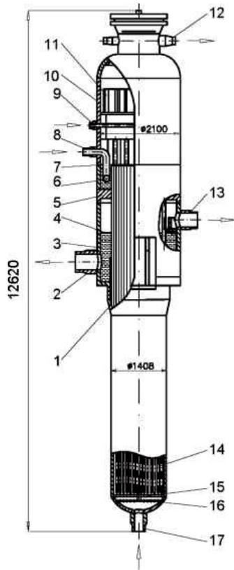
Рис. 4.20. Испаритель (а) и труба Фильда (б) паро-генератора БН-350: 1 - корпус испарителя;
