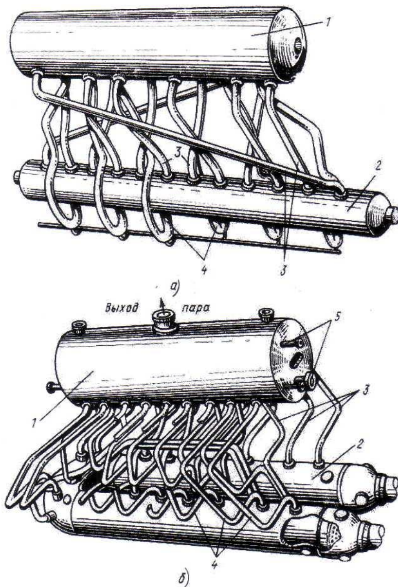
Рис. 4.11. Паро- генераторы АЭС «Шип- пингпорт»: А - с прямыми и б - с U-образны- ми трубками
