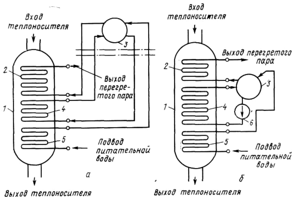
Рис. 4.31. Схема парогенераторов со змеевиковыми поверхностями обмена: а - с естественной циркуляцией и б - с многократной циркуляцией: 1 - корпус ПГ; 2- пароперегреватель; 3-сепарационный барабан; 4 - испаритель; 5 - водяной экономайзер; 6 - насос тельной циркуляции
