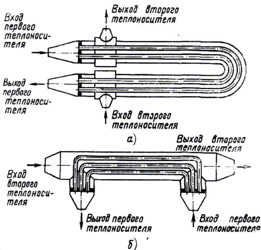
Рис. 4.4. Теплообменники:
