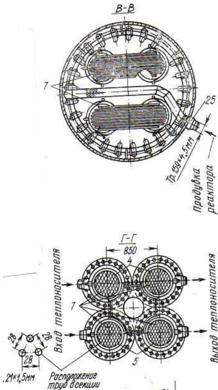
Рис. 4.10. ПГ установки НИИАР. Виды В-В и Г-Г.
