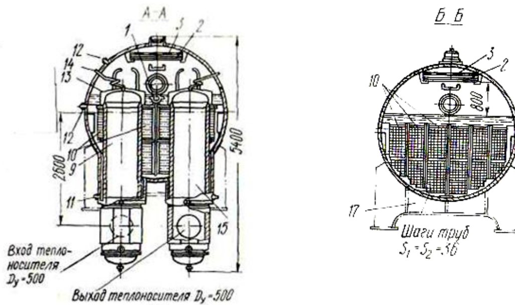
Рис. 4.7. Парогенератор I блока НВАЭС. Вид А-А и Б-Б. Обозначения как на рис. 4.6
