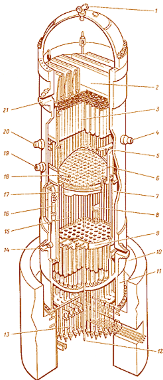
Рис. 3.12. Конструкция реактора с кипящей водой BWR на АЭС «Grand Gulf» (США):
