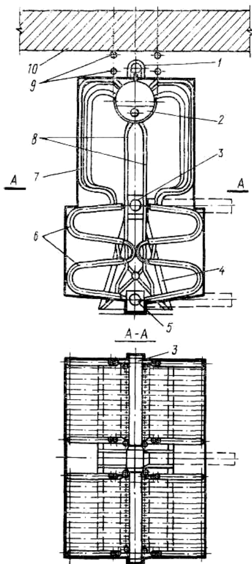
Рис. 4.13. Схема секционного ПГ:
