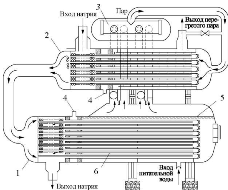
Рис. 4.15. Парогенератор
