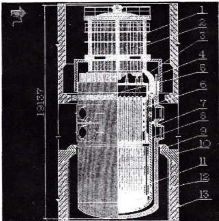
Рис. 3.1. Реактор ВВЭР-1000:
