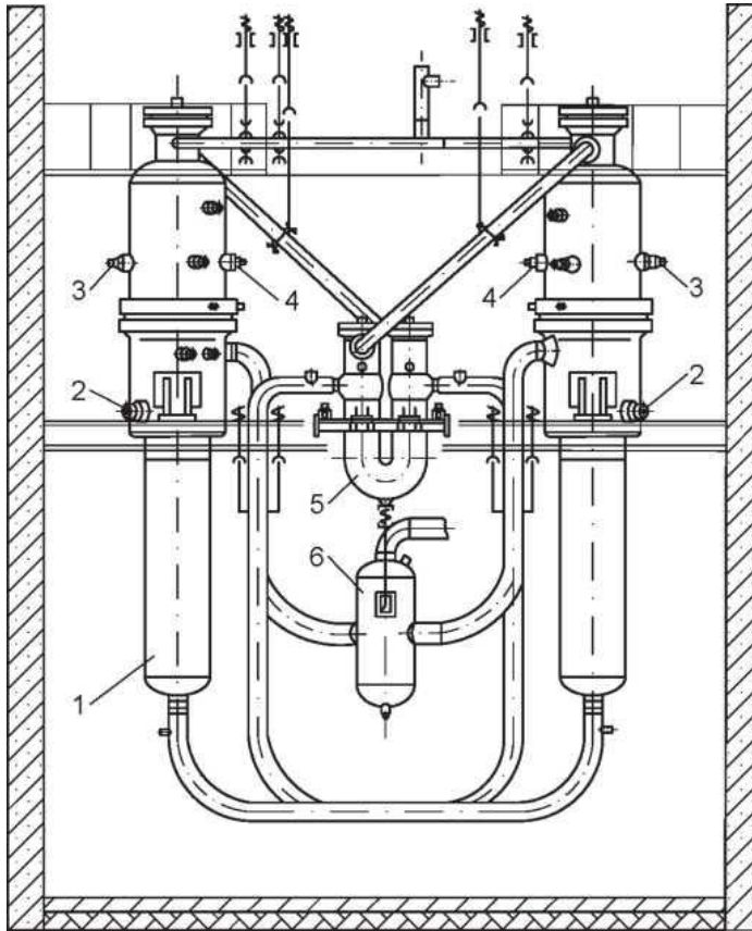
Рис. 4.19. Компоновка ПГ РУ БН-350:
