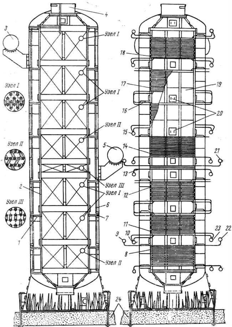
Рис. 4.32. ПГ АЭС «Колдер-Холл»: 1- площадка; 2- кожух; 3- сепарационный барабан повышенного давления; 4- подводящий патрубков; 5- сепарационный барабан низкого давления; 6- лестница; 7- корпус; 8- смешанный экономайзер; 9- выходной коллектор части повышенного давления смешанного экономайзера; 10- входной коллектор испарителя низкого давления; 11,12- нижний и верхний пакеты испарителя низкого давления; 13- пароперегреватель низкого давления; 14- экономайзер повышенного давления; 15- входной коллектор испарителя повышенного давления; 16,17- нижний и верхний пакеты испарителя повышенного давления; 18- пароперегреватель повышенного давления; 19- обшивка ПГ; 20- люк; 21- выходной коллектор пароперегревателя низкого давления; 22- входной коллектор испарителя низкого давления; 23- выходной коллектор части низкого давления смешанного экономайзера; 24- бетонный фундамент
