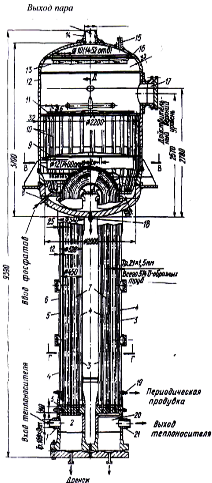
Рис. 4.9. ПГ установки НИИАР: 1, 21- патрубки входа и выхода теплоносителя;
