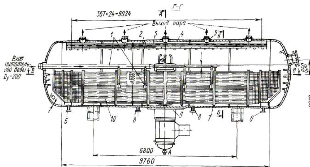
Рис. 4.6. Парогенератор I блока НВАЭС. Вид Г-Г: 1 - труба подачи питательной воды; 2- жалюзийный сепаратор; 3-пароприемный потолок; 4- корпус; 5 - паропроводящие трубы; 6, 8 - штуцера непрерывной и периодической продувки; 7 - опоры трубок; 9 - входной коллектор; 10 - поверхность теплообмена; 11- штуцера дренажа; 12- штуцера уровнемеров; 13 - защитный кожух; 14 - воздушники; 15- выходной коллектор теплоносителя; 16 - опорные скобы; 17 - опоры
