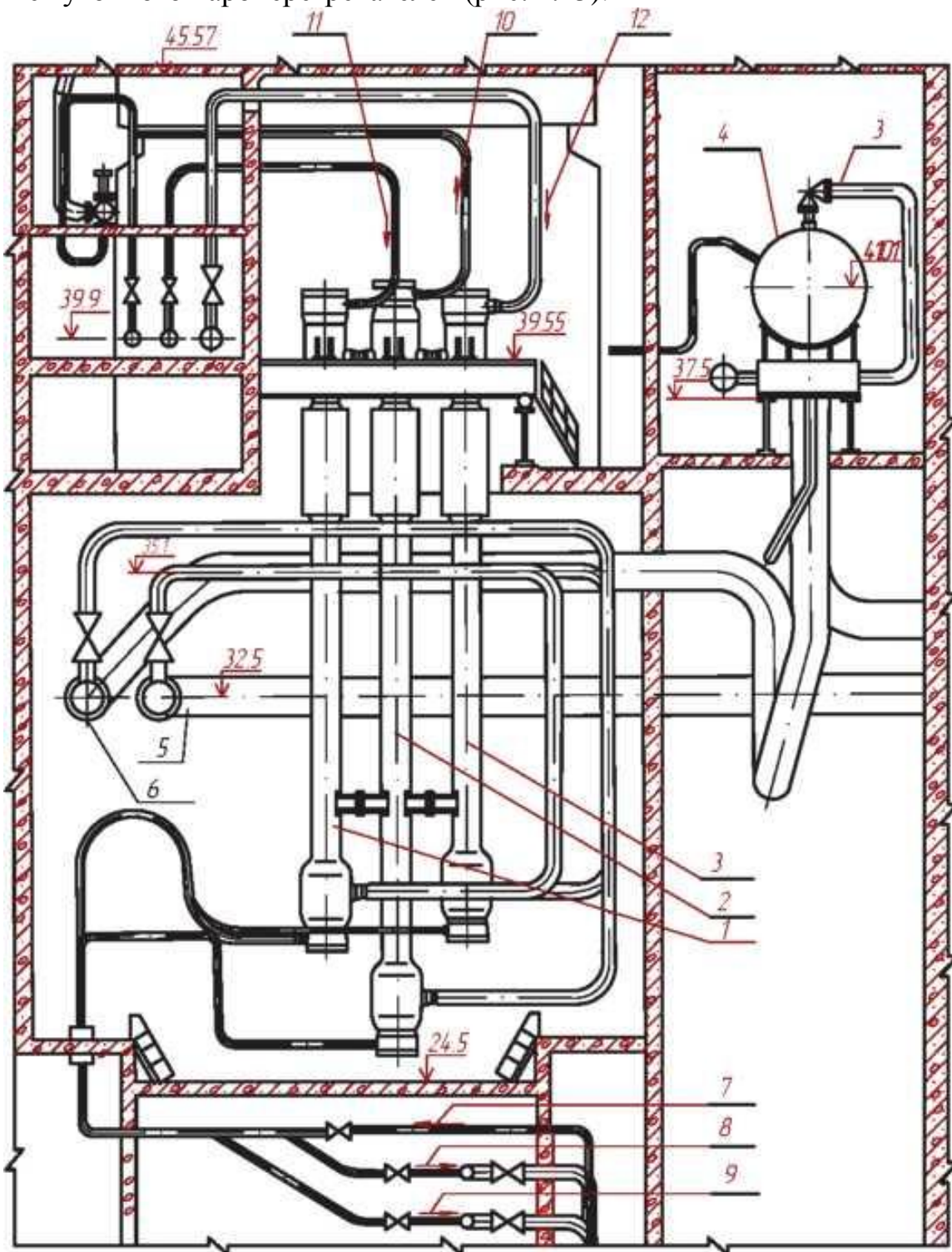
Рис. 4.23. Компоновка парогенератора в боксе: 1 - пароперегреватель; 2 - испаритель; 3 - промпароперегреватель; 4 - буферная емкость; 5 - подвод натрия; 6 - отвод натрия; 7 - подвод питательной воды; 8 - отвод пара промперегрева; 9 - отвод острого пара; 10 - отвод слабоперегретого пара; 11 - подвод пара к пароперегревателям; 12 - подвод пара промперегрева [10]
