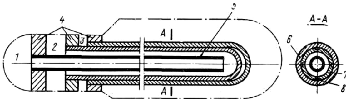
Рис. 4.21. Схема поверхности теплообмена из обратных элементов с двойными наружными трубками: 1 - входная камера теплоносителя; 2 - выходная камера теплоносителя; 3 - камера инертного газа; 4 - трубные доски; 5 - обратная трубка; 6 - наружная трубка; 7 - внутренняя трубка; 8 - каналы, заполненные инертным газом
