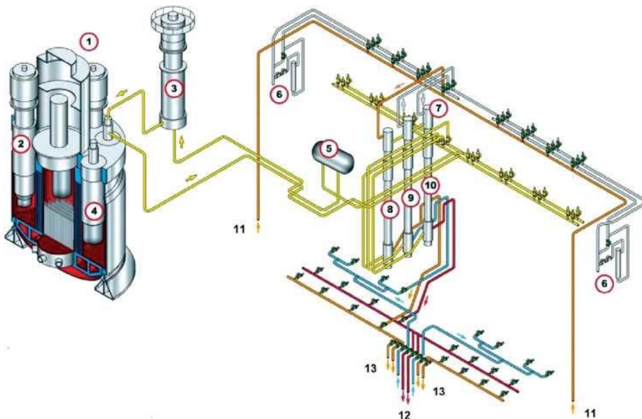
Рис. 4.24. Компоновка парогенератора ПГН-200М в составе реакторной установки БН-600: 1 - реактор; 2 - ГЦН-I; 3 - ГЦН-II; 4 - промежуточный теплообменник; 5 - буферная емкость; 6 - растопочный сепаратор; 7 - модули парогенератора; 8 - промпароперегреватель; 9 - испаритель; 10 - основной пароперегреватель; 11 - пар после ЦВД; 12 - пар на ЦВД; 13 - пар на ЦСД
