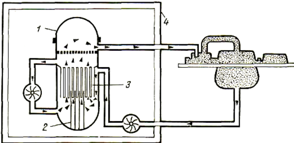
Рис. 3.11. Кипящий реактор с легководным замедлителем и теплоносителем (BWR): 1- стальной корпус давления; 2 – регулирующие стержни; 3 – топливные элементы; 4 - бетонная защита
