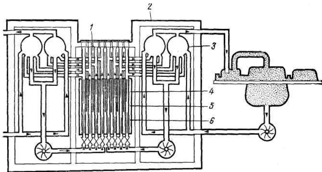
Рис.3.7. Тепловая схема кипящего легководного реактора с графитовым замедлителем РБМК: 1- регулирующие стержни; 2 - бетонная защита; 3 - паровые барабаны; 4 - графитовый замедлитель; 5 - трубки давления; 6 - топливные элементы
