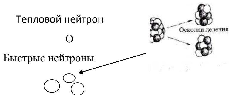
Рис. 2.2. Схема деления ядер урана-235
