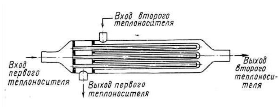
Рис. 4.3. Теплообменник с обратными элементами
