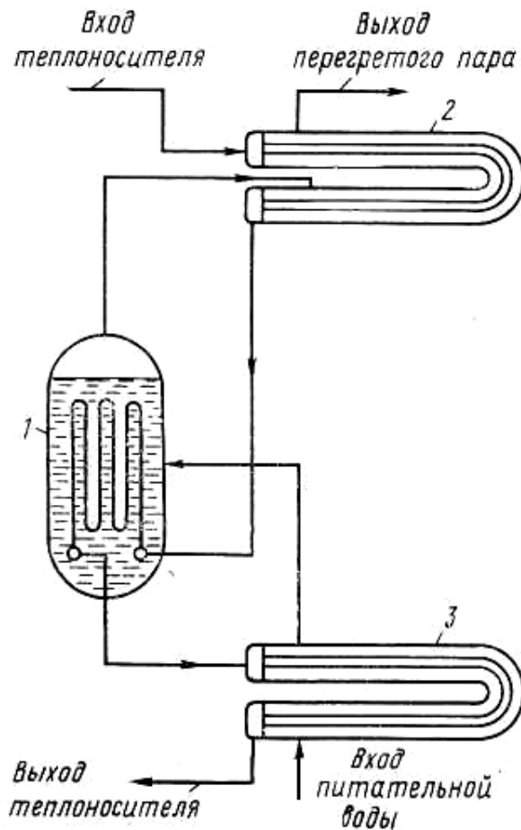
Рис. 4.5. Принципиальная схема ПГ Первой (Обнинской) АЭС:
