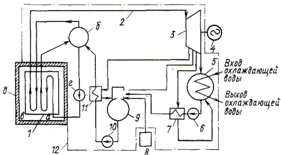
Рис. 3.2. Принципиальная схема одноконтурной АЭС: 1- ядерный реактор; 2- паропровод; 3 - паровая турбина; 4- электрогенератор; 5 - конденсатор; 6 - конденсатный насос; 7 - подогреватель воды низкого давления; 8 - установка для подготовки добавочной воды; 9 - деаэратор; 10 - питательный насос; 11 - подогреватель воды высокого давления; 12 - биологическая защита паротурбинного контура; а - испарительная часть реактора; б - сепарационный барабан; в - пароперегревательная часть реактора; г - перекачивающий насос; д - биологическая защита реактора
