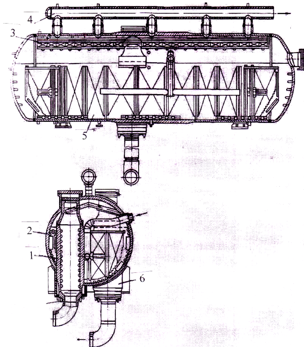
Рис. 4.12. ПГ III блока НВАЭС: 1 - входной коллектор теплоносителя; 2 - корпус ПГ; 3 - жалюзийный сепаратор; 4 - коллектор сухого пара; 5 - поверхность теплообмена; 6 - выходной коллектор теплоносителя
