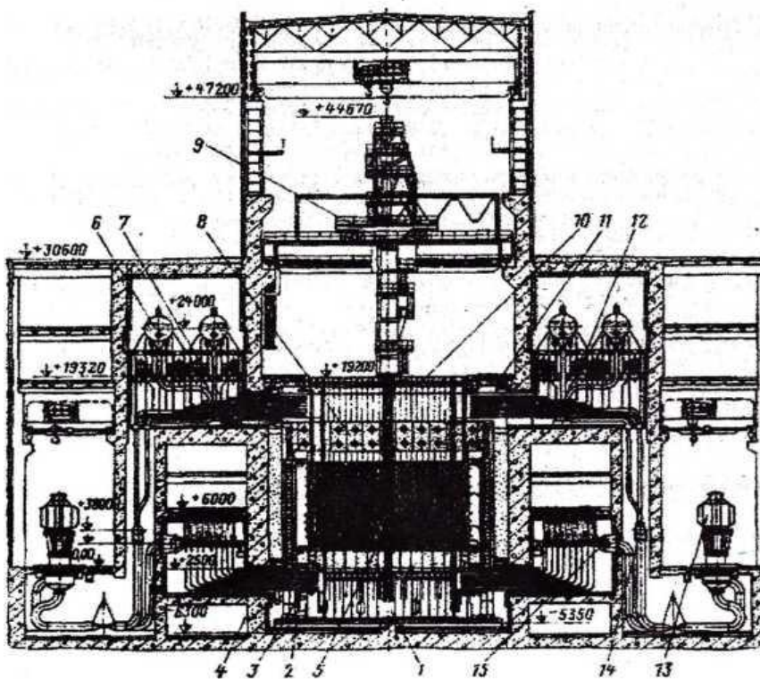
Рис 3.6. Общий вид реактора РБМК:
