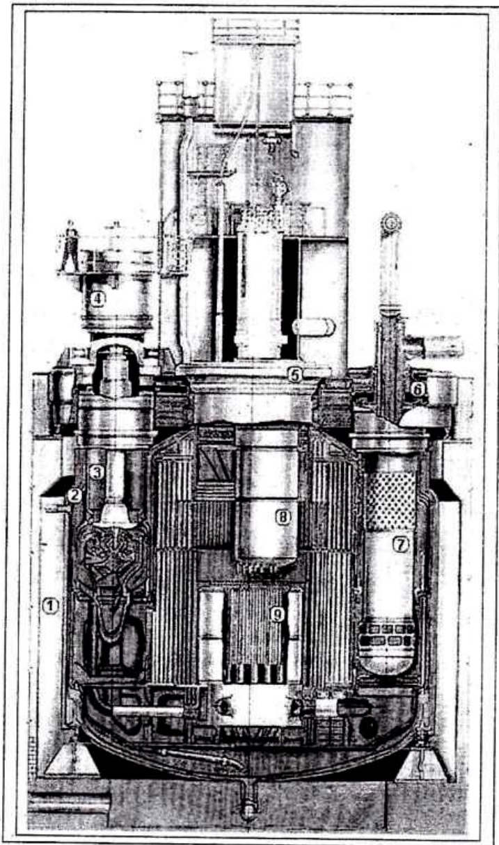
Рис. 3.16. Реактор БН-600 [6]:
