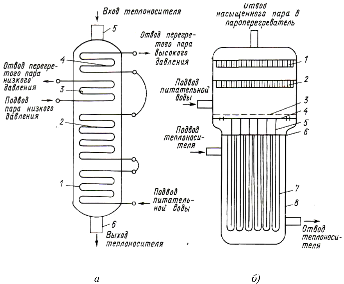
Рис. 4.30. Схема прямоточного ПГ с промежуточным пароперегревателем: а - 1- экономайзер; 2 - испаритель; 3- промежуточный пароперегреватель; 4- пароперегреватель высокого давления; 5,6 - патрубки подвода и отвода теплоносителя и схема испарителя с поверхностью теплообмена из «обратных элементов»; б - 1- вторая ступень механической сепарации; 2 - первая ступень механической сепарации; 3 - погруженный дырчатый щит; 4 - трубная доска внутренних трубок; 5,7 – внутренняя и внешняя трубки элемента; 6 - трубная доска внешних трубок; 8 — корпус
