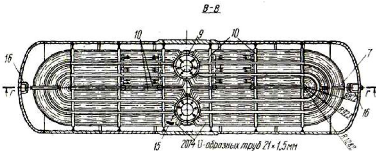
Рис. 4.8. Парогенератор I блока НВАЭС. Вид В-В. Обозначения как на рис. 4.6
