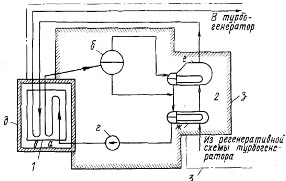
Рис. 3.3. Принципиальная схема производства рабочего пара на 1-м блоке Белоярской АЭС им. И. В. Курчатова: 1- ядерный реактор: а- испарительная часть реактора; б - разделительный (сепарационный барабан); в - пароперегревательная часть реактора; г - перекачивающий насос реактора; д - биологическая защита реактора; 2 - парогенераторная установка: е - испаритель ПГ; ж - подогреватель (водяной экономайзер) ПГ; з - биологическая защита ПГ; 3 - биологическая защита паротурбинного контура
