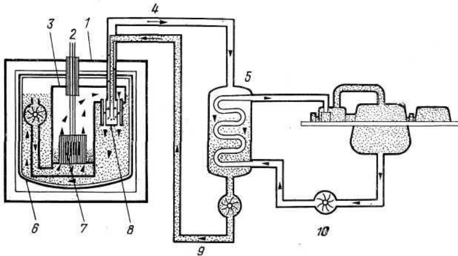
Рис. 3.15. Схема быстрого реактора с натриевым теплоносителем:
