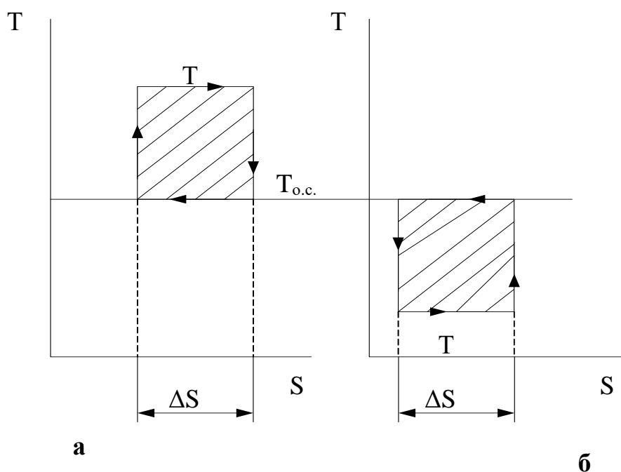
Рис. 4.2. Циклы Карно: а – прямой, б – обратный
