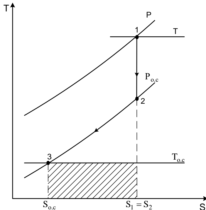
Рис. 4.4. Схема обратимого взаимодействия потока вещества с окружающей средой
