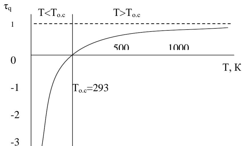
Рис.4.3. Зависимость \tau_q от T
