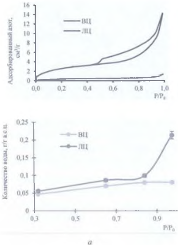
Рис. 5. Кривые адсорбции (а) - десорбции (б) паров воды водорослевой и лиственной целлюлозы
