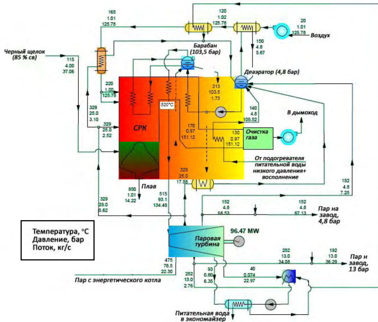
Рис. П2.3. Тепловой и материальный балансы системы регенерации химикатов с использованием СРК Производительность 1580 т асц/сут [26]
