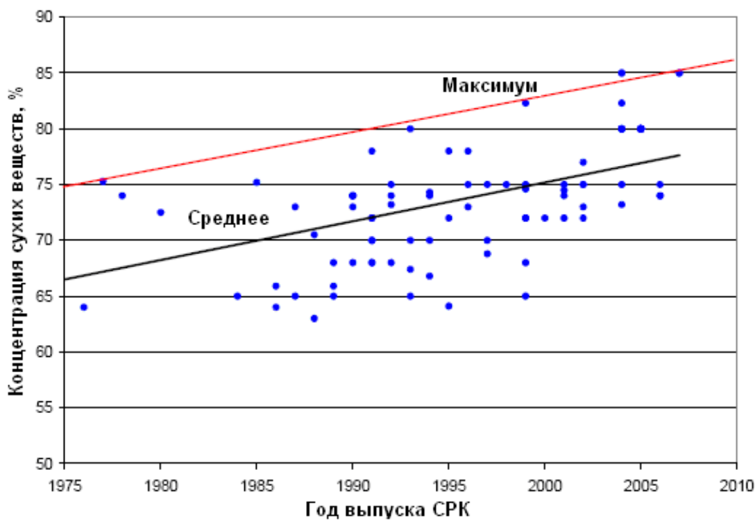
Рис. П1.1. Изменение концентрации сухих веществ черного щелока в зависимости от года выпуска СРК [21]
