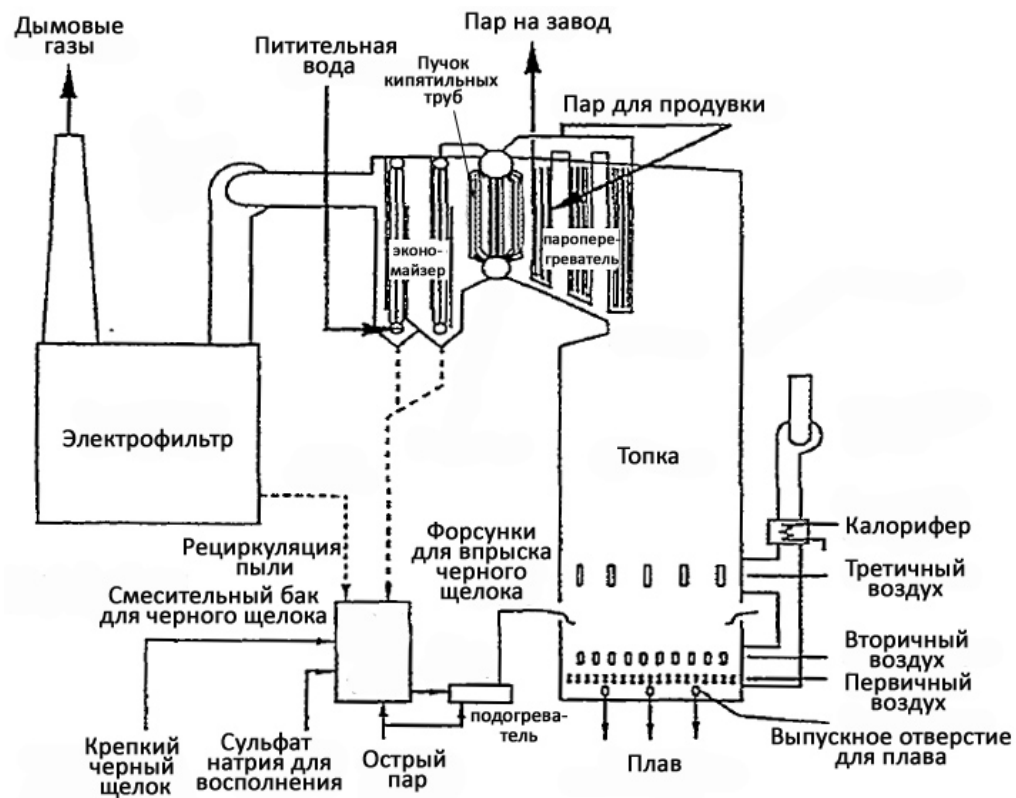
Рис. 5. Устройство двухбарабанного СРК
