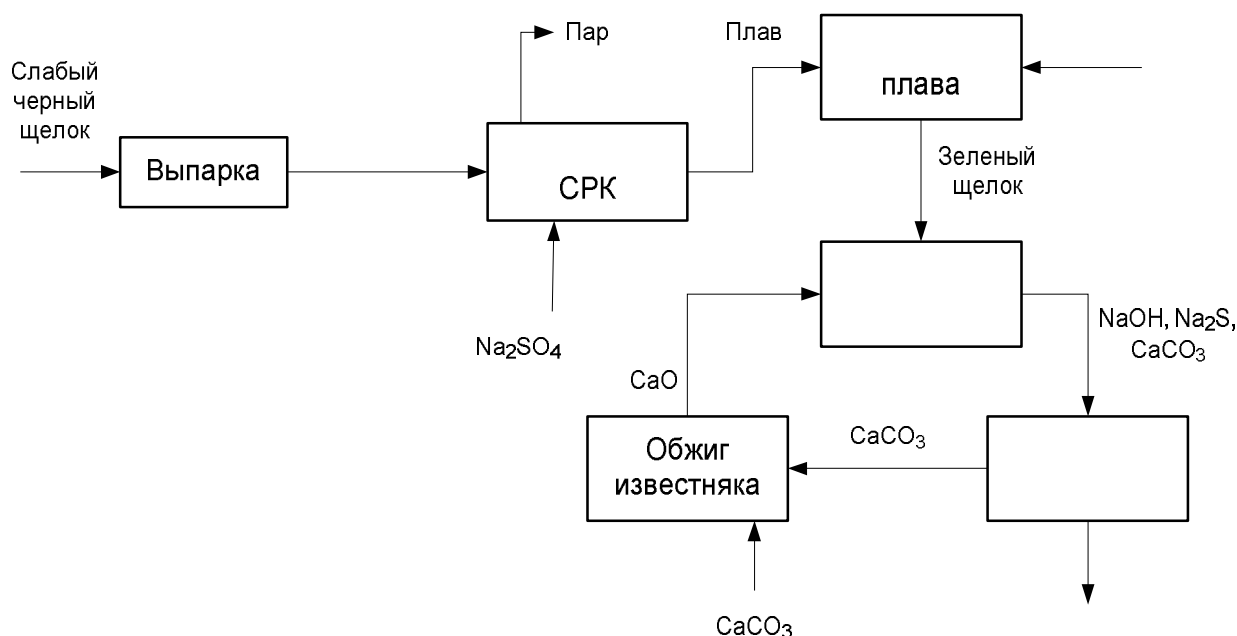
Рис. 2. Система регенерации химикатов
