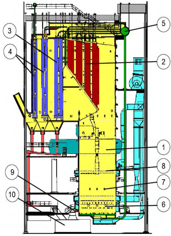
Рис. 7. Устройство современного СРК: 1-топка; 2-пароперегреватель; 3-пучок кипящих труб; 4-экономайзер; 5-однотрубный паровой котел; 6-входные отверстия первичного и вторичного воздуха; 7-форсунка подачи шлока; 8-подача третичного воздуха; 9-выпускные отверстия плава; 10-бак растворения плава
