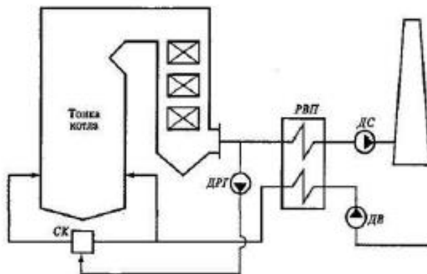
Рис. 1. Рециркуляция дымовых газов: ДРГ – дымосос рециркуляции газов; РВП - ...
