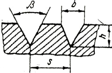
Рис.2.5. Конфигурация поверхности дефибрерного камня после насечки
