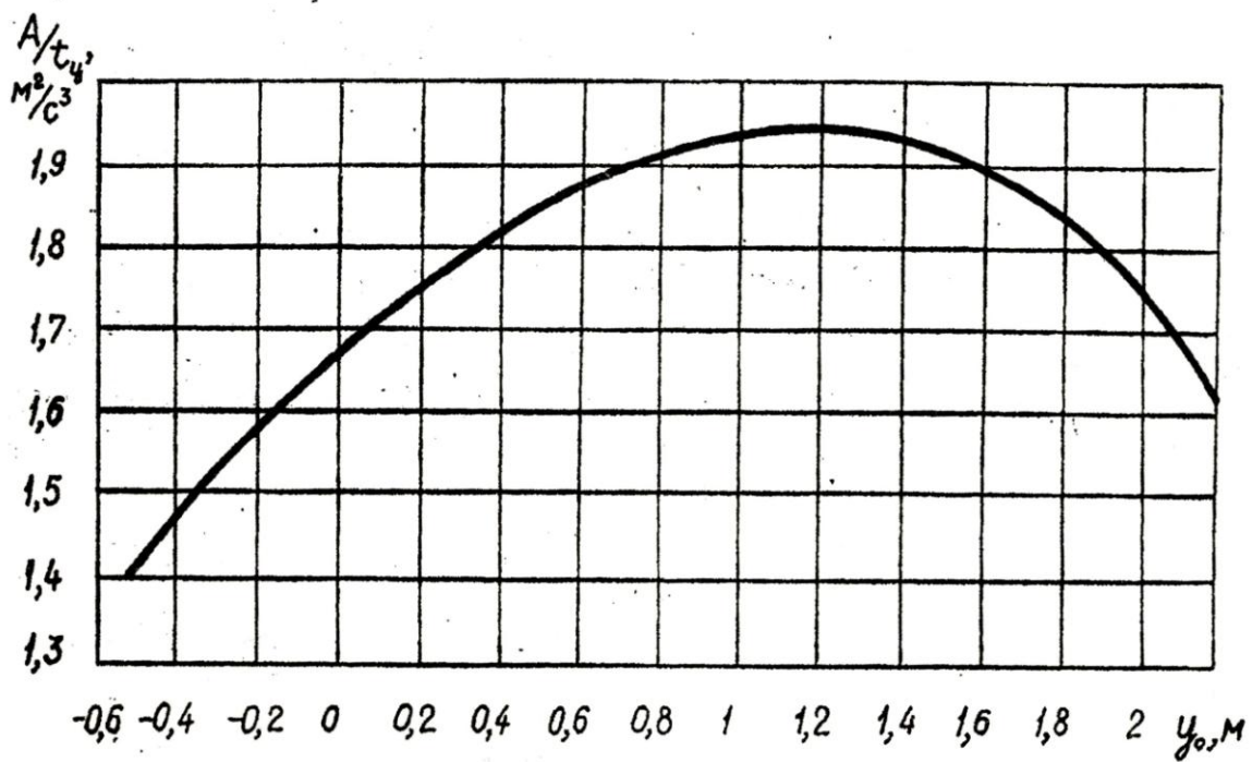
Рис. 1.10. Зависимость \dot{A}t_{\delta}^{-1} = f(y_o) для барабана диаметром 3,85 м при \omega = 0,28 \omega_{кр}
