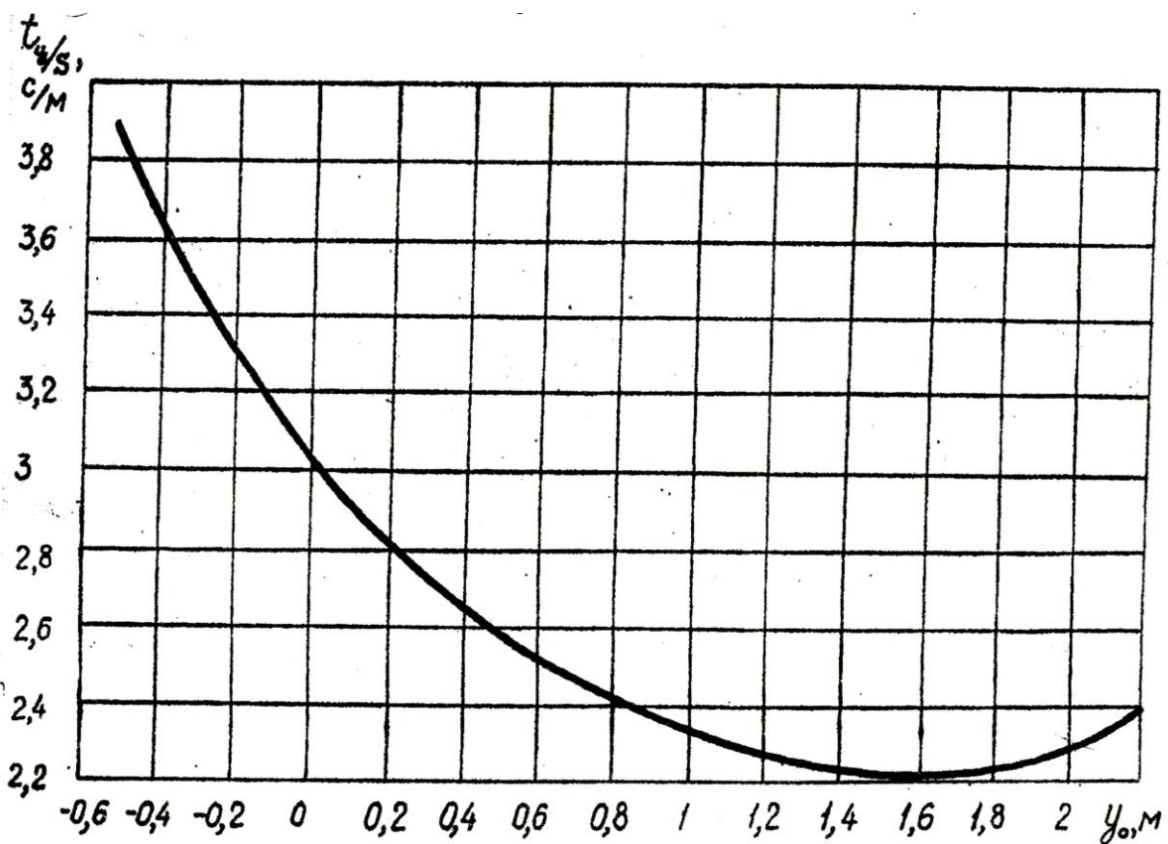
Рис. 1.9. Зависимость t_w S^{-1} = f(y_o) для барабана диаметром 5 м при \omega = 0,28 \omega_{кр}
