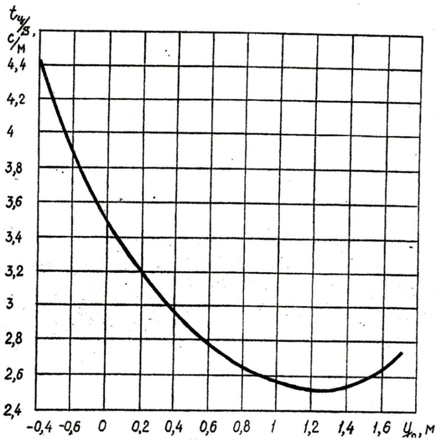
Рис. 1.8. Зависимость t_w S^{-1} = f(y_o) для барабана диаметром 3,85 м при \omega = 0,28 \omega_{кр}
