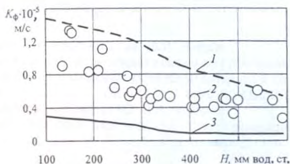
Рис. 2. Изменение коэффициента фильтрации K_{\phi} в зависимости от приложенного напора H для газетной бумаги: 1 – с минимальной аэрацией, 2 – по обычной методике, 3 – с максимальной аэрацией
