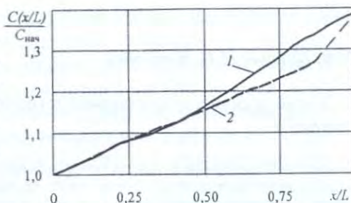
Рис. 1. Изменение относительной сухости C(x/L) / C_{нач} бумажной массы в зависимости от относительной длины x/L участка формирования сеточного стола с гидропланками: 1 – расчет, 2 – эксперимент ( C_{нач} – сухость бумажной массы перед первой гидропланкой)
