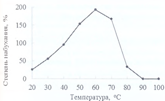
Рис. 4. Зависимость степени набухания пленки от различной температуры
