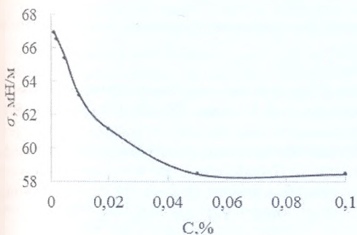
Рис. 6. Зависимость поверхностного натяжения от концентрации агара в растворе
