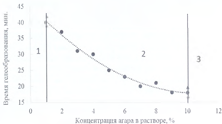
Рис. 3. Зависимость времени гелеобразования от концентрации агара в растворе при температуре 25 °С
