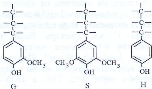
Рис. 1. Фенилпропановые единицы лигнина: G - гваяцилпропановый тип, S-сирингилпропановый тип, H - п-кумаровый тип
