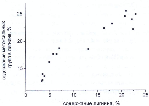
Рис. 5. Зависимость содержания метоксильных групп в лигнине от содержания лигнина в образцах
