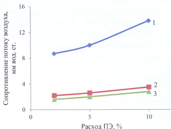
Рис. 6. Зависимость сопротивления потоку воздуха от расхода ПЭ для волокон: 1 – МТВ-0,25; 2 – МТВ-0,40; 3 – УТВ-0,60
