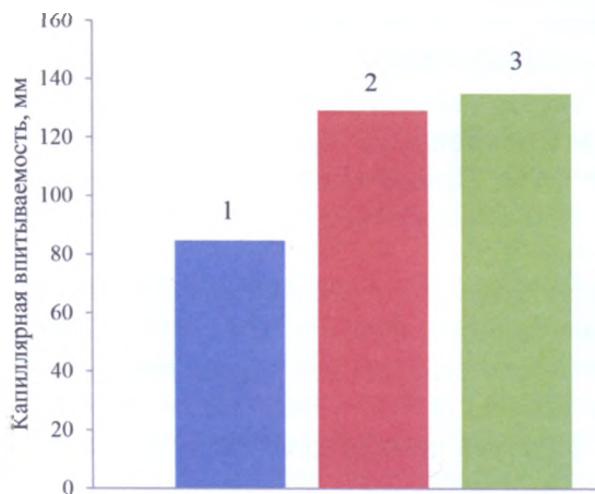
Рис. 2. Капиллярная впитываемость при расходе ПВА 10 % для волокон: 1 – МТВ-0,25; 2 – МТВ-0,40; 3 – УТВ-0,60
