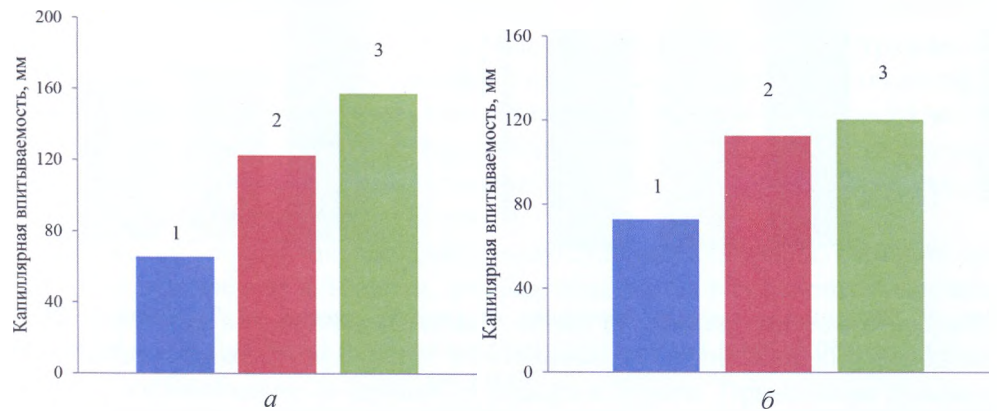
Рис. 11. Зависимость капиллярной впитываемости от расхода смесей 40 % ТММ + 20 % Al_2(SO_4)_3 (а) и 50 % ТММ + 10 % Al_2(SO_4)_3 (б) для волокон: 1 – МТВ-0,25; 2 – МТВ-0,40; 3 – УТВ-0,60
