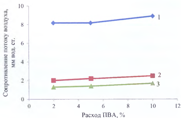
Рис. 3. Влияние расхода ПВА на сопротивление потоку воздуха для волокон: 1 – МТВ-0,25; 2 – МТВ-0,40; 3 – УТВ-0,60
