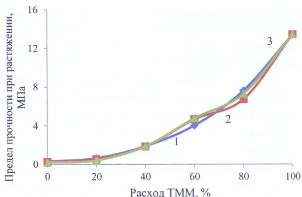
Рис. 7. Зависимость предела прочности при растяжении от расхода ТММ для волокон: 1 – МТВ-0,25; 2 – МТВ-0,40; 3 – УТВ-0,60
