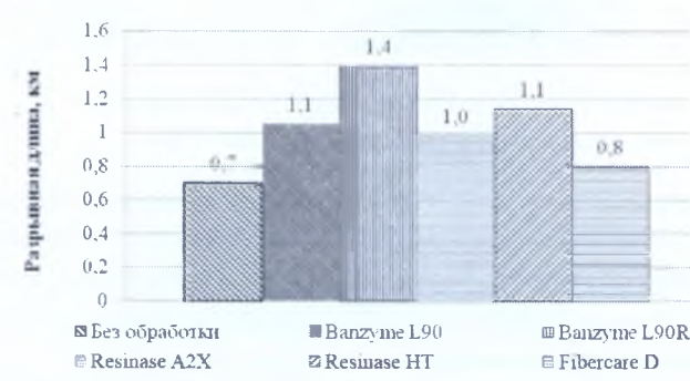
Рис. 1. Влияние ферментативной обработки на разрывную длину отливок из волокон ХТММ из древесины Larix sibirica Ledeb (Pinaceae)
