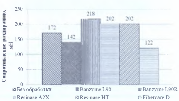
Рис. 2. Влияние ферментативной обработки на сопротивление раздиранию отливок из волокон ХТММ из древесины Larix sibirica Ledeb (Pinaceae)
