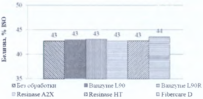
Рис. 3. Влияние ферментативной обработки на белизну волокон ХТММ из древесины Larix sibirica Ledeb (Pinaceae)
